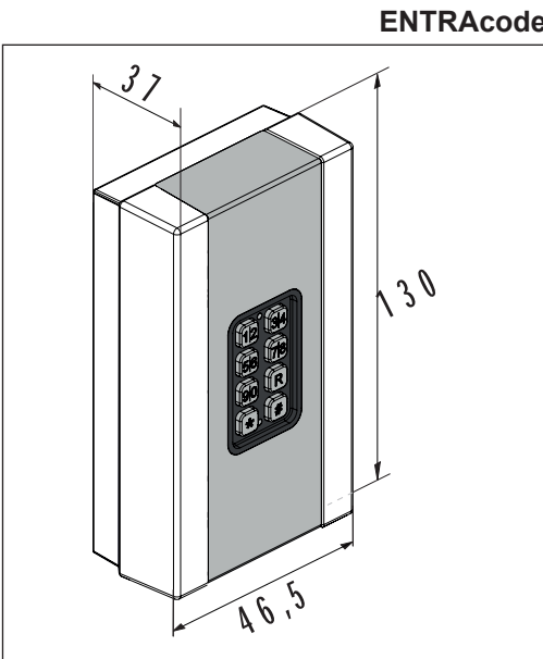
Abb. Abmessungen ENTRAcod+ AP (alle Angaben in mm)
