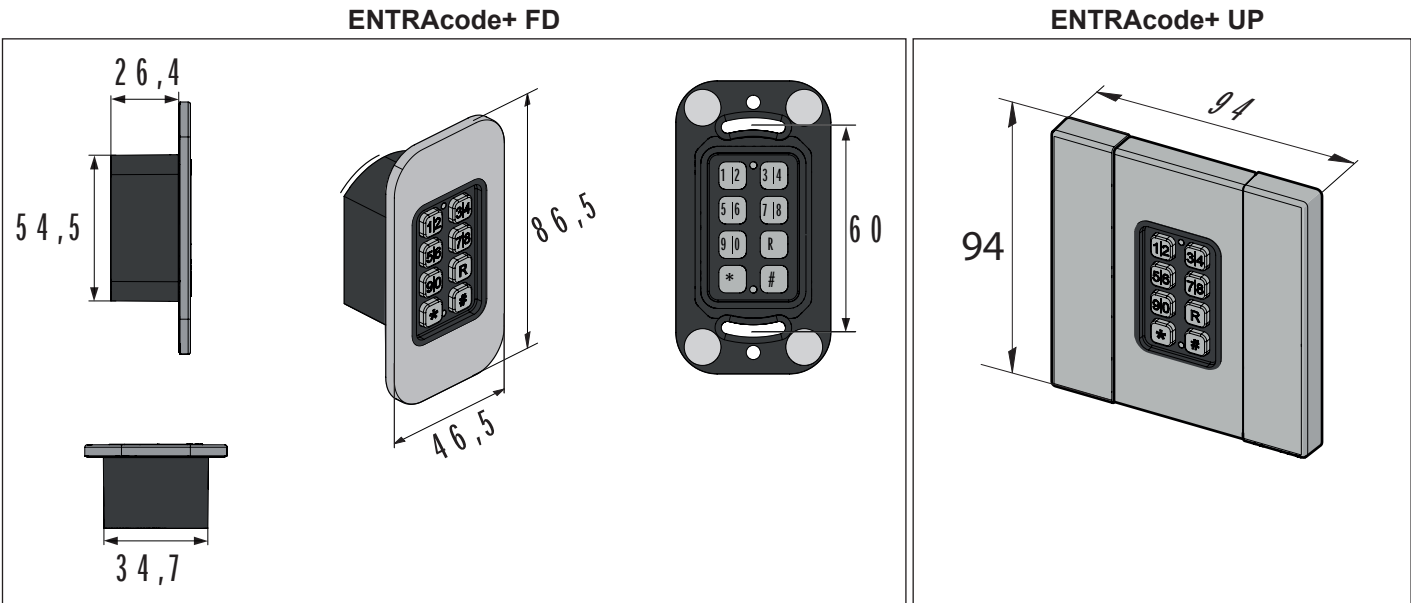
Abb. Abmessungen ENTRAcod+ FD / UP (alle Angaben in mm)
