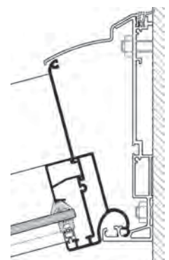
Wandanschluss- Schwenk
