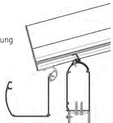
Dachüberstand Stützenbefestigung
