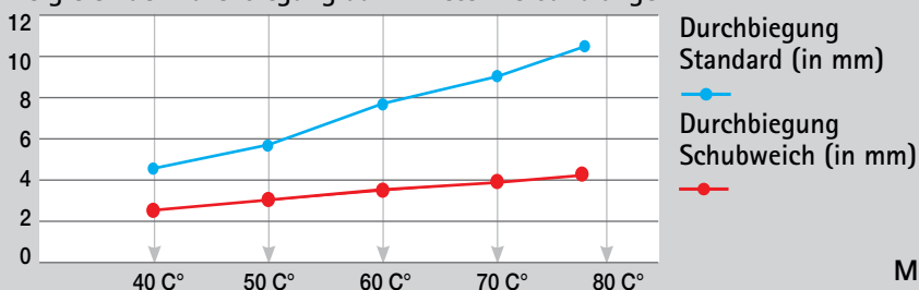
Vergleich der Durchbiegung auf 2 Meter Verbundlänge
